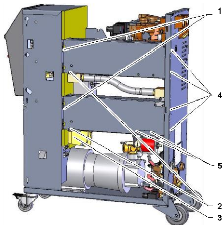
Sl. 79: demontaža gretja
