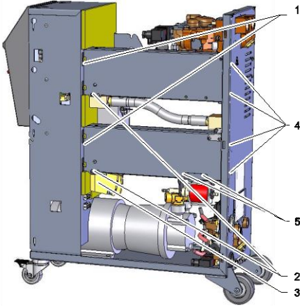
Рис. 78: Демонтаж термоэлемента
