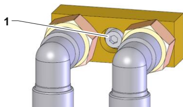
Рис. 12: центральное крепление
