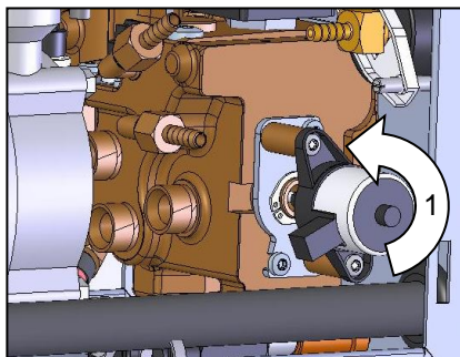
Afb. 80: Koelklep 1 demonteren
