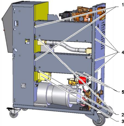
Afb. 79: Verwarming demonteren
