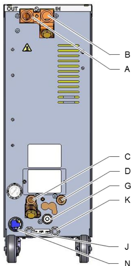
Afb. 5: Aansluitingen
