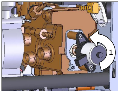
Afb. 76: Koelklep 1 demonteren
