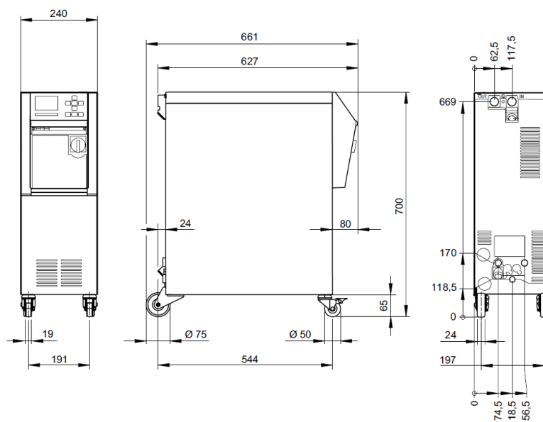
Afb. 2: Afmetingen
