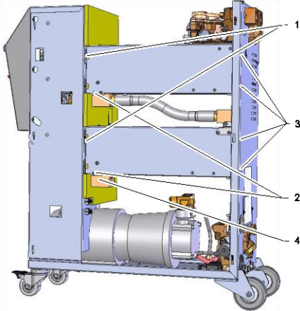
Ábra 75: Fűtés kiszerelése
