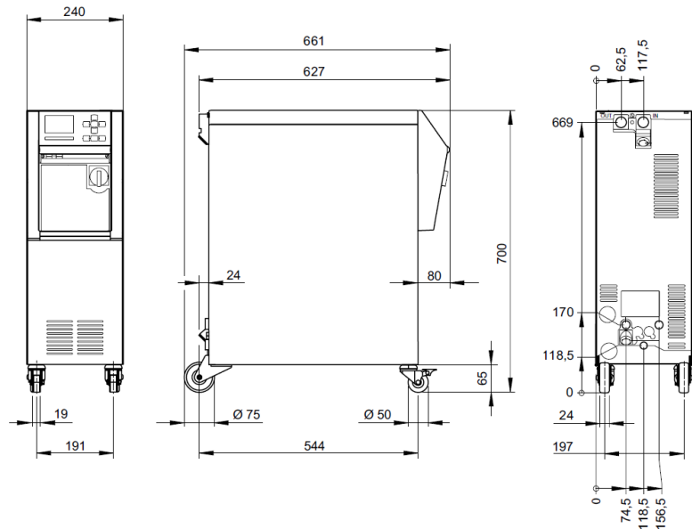
Ábra 2: Méretek
