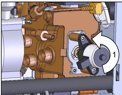
Ábra 76: Hűtőszelep 1 kiszerelése
