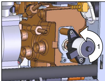
Abb. 76: Kühlventil 1 ausbauen
