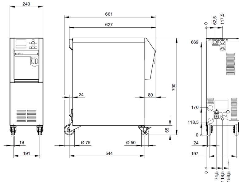
Abb. 2: Abmessungen
