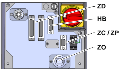
Abb. 13: Schnittstellen Panel-5
