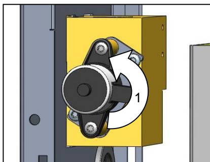
Bild 77: Demontera kylventil 1
