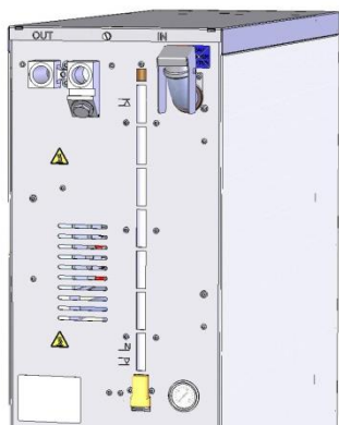
Рис. 11: Заполнение устройства
