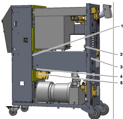
Рис. 76: Демонтаж термоэлемента
