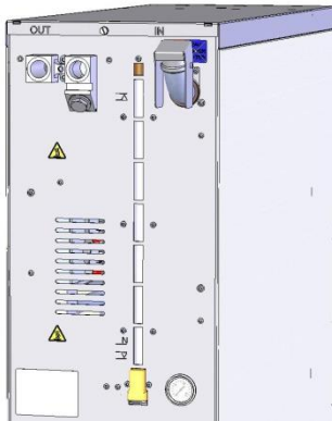
Fig. 11: Remplissage du thermorégulateur
