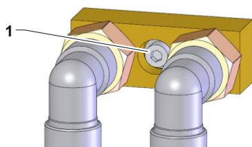
Fig. 10: Fixation centrale
