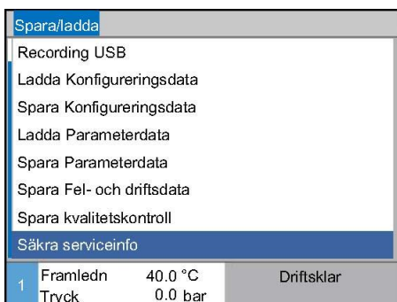
Bild 62 Spara data
