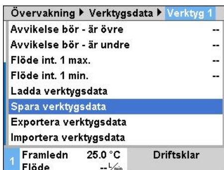
Bild 64: Spara verkytsdata
