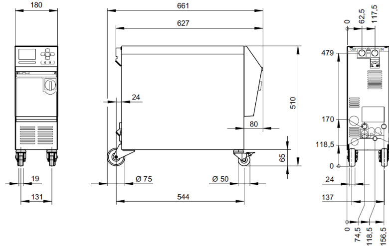
Afb. 2: Afmetingen
