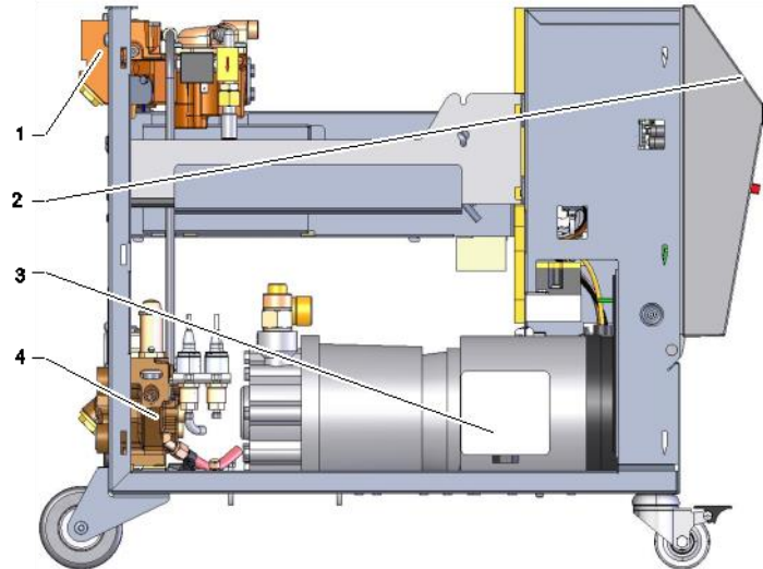
Afb. 4: Overzicht
