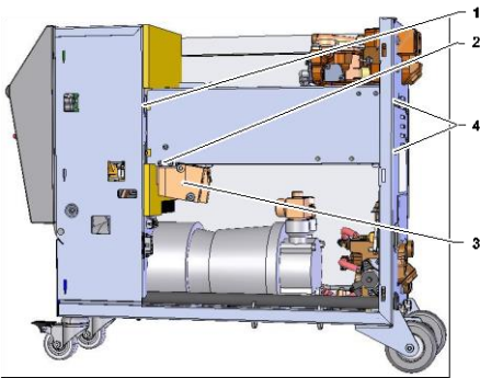
Afb. 75: Verwarming demonteren
