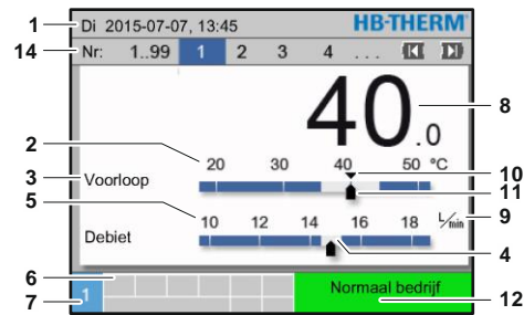
Afb. 18: Basisaanduiding Graph
