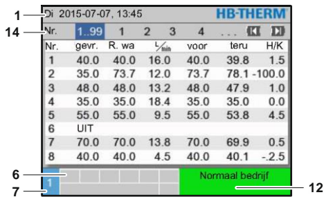
Afb. 17: Basisaanduiding Tabel
