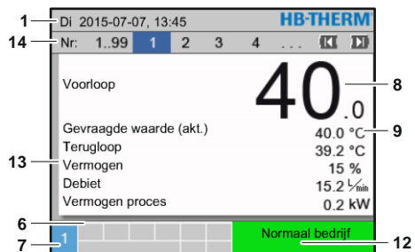
Afb. 19: Basisaanduiding Text
