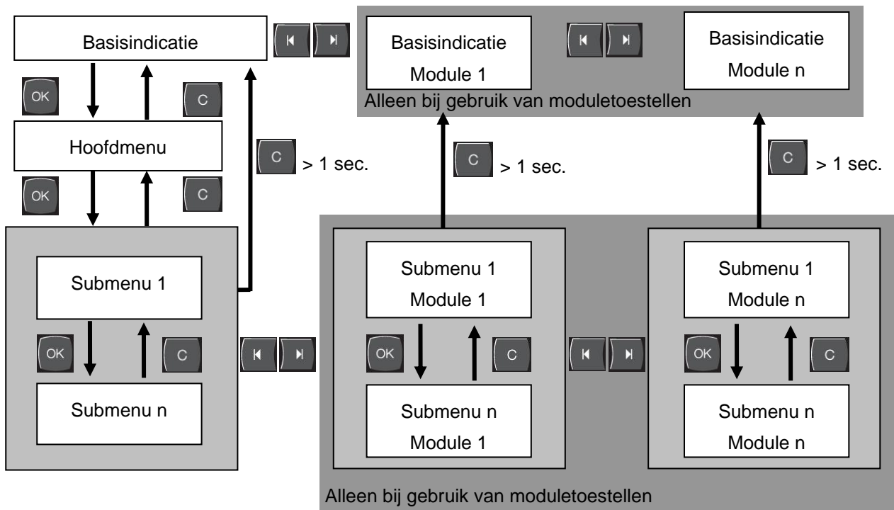
Afb. 21: Bedieningsstructuur
