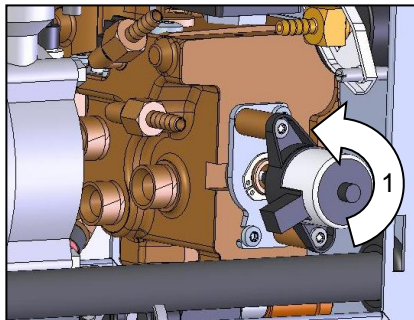
Afb. 76: Koelklep 1 demonteren
