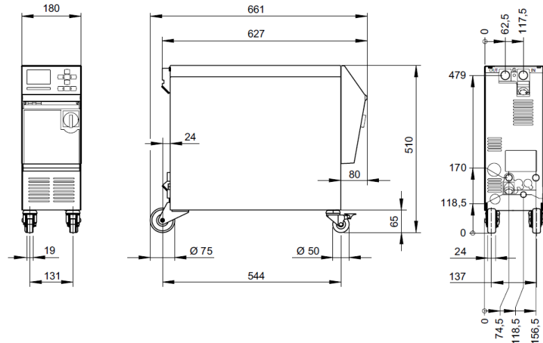
Fig. 2 : Dimensions
