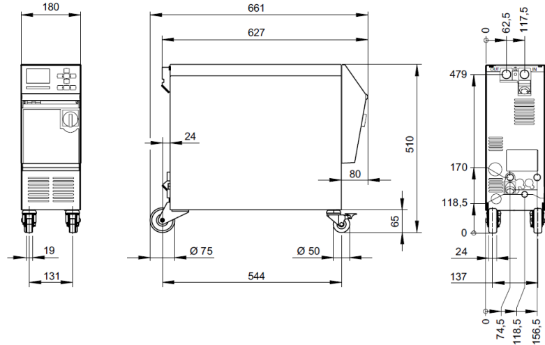
Fig. 2: Dimensiones
