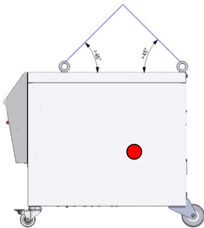
Abb. 7: Anschlagpunkte
