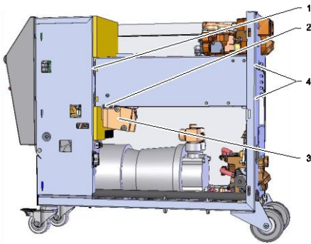
Abb. 75: Heizung ausbauen
