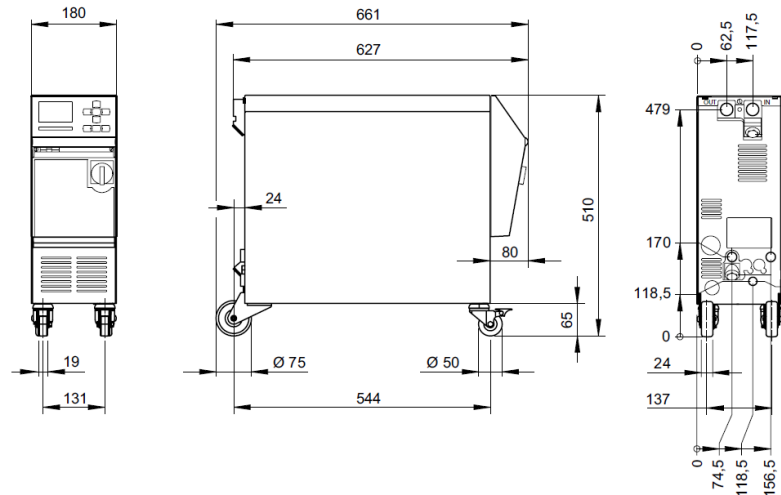
Abb. 2: Abmessungen
