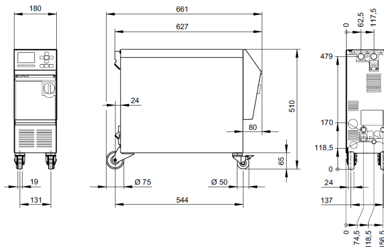
Фиг. 2: Размери
