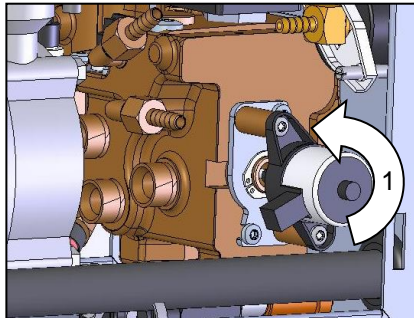
Sl. 78: demontaža hladilnega ventila 1
