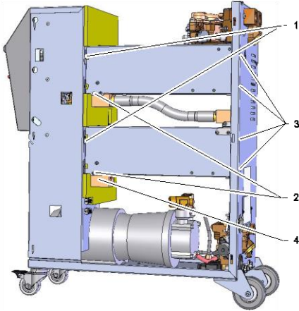
Sl. 77: demontaža gretja
