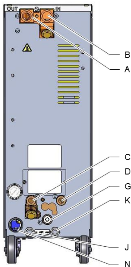
Рис. 5: Подключения
