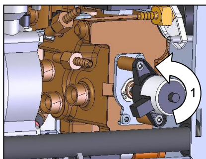
Рис. 78: Демонтаж клапана линии охлаждения 1
