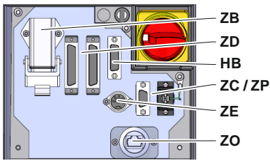
Abb. 11: Schnittstellen Einzelgerät
