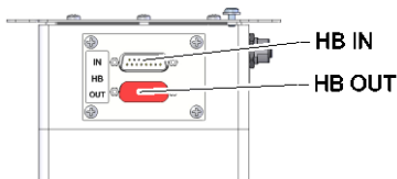
Abb. 15: Schnittstellen Flow-5 Bauart: Autonom
