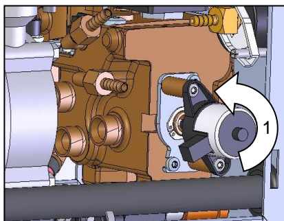
Abb. 78: Kühlventil 1 ausbauen
