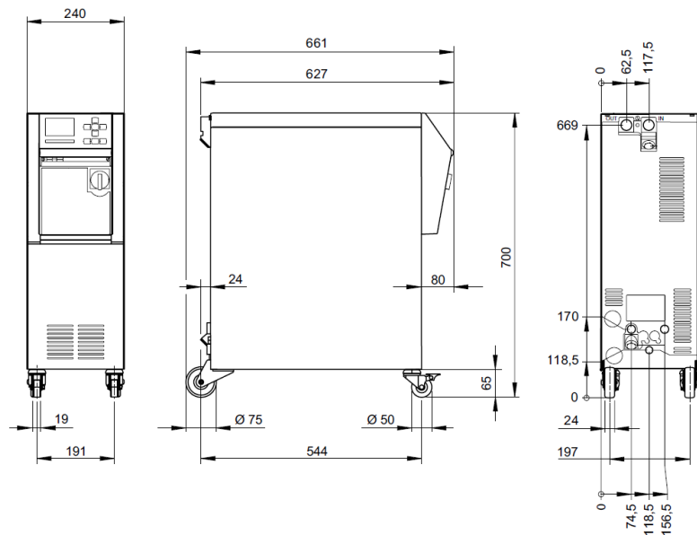
Abb. 2: Abmessungen
