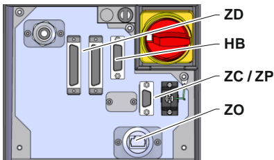
Abb. 13: Schnittstellen Panel-5
