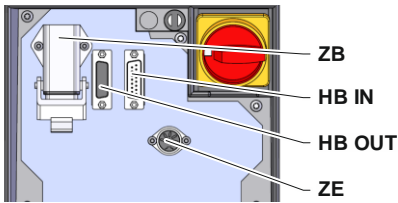
Abb. 12: Schnittstellen Modulgerät
