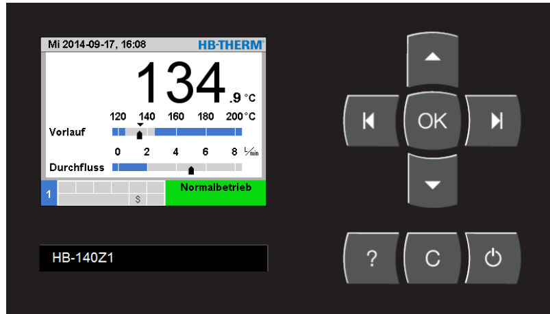
Abb. 18: Tastatur und Anzeige
