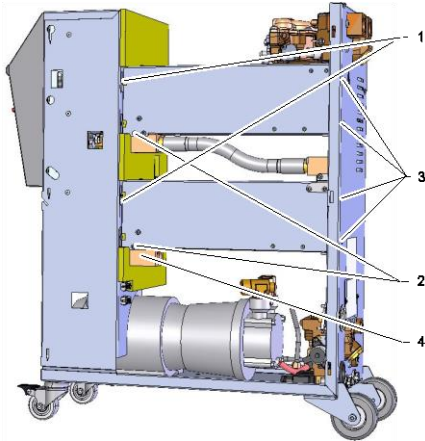
Ill. 77: Afmonter varmesystemet
