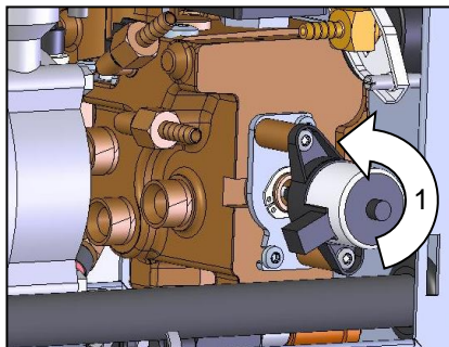
Ill. 78: Afmonter køleventil 1
