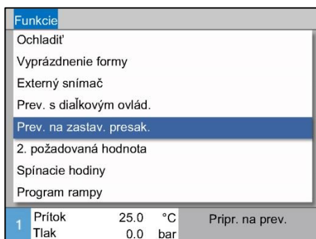
Obr. 35: Zapnutie prevádzky na zastavenie presakovania
