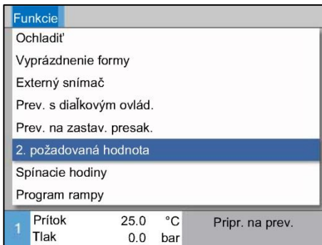
Obr. 40: Nastavenie 2. požadovanej hodnoty
