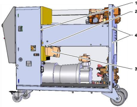
Bild 77: Demontera uppvärmningen
