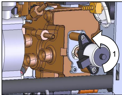
Bild 78: Demontera kylventil 1
