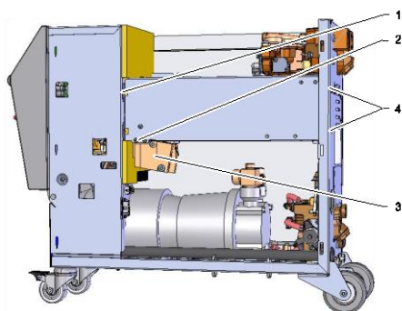
Fig. 77 : Déposer le chauffage
