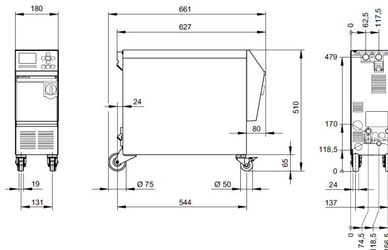
Fig. 2 : Dimensions
