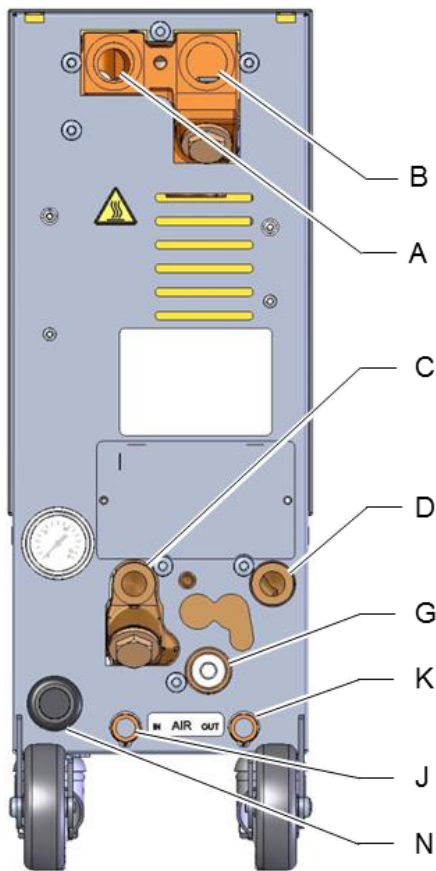
Fig. 5 : Raccords
