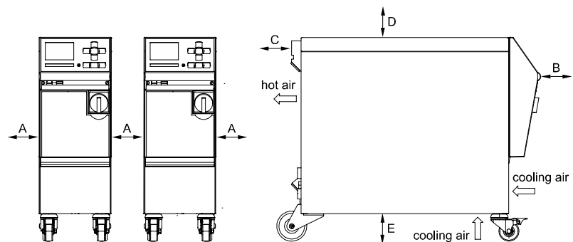
fig. 3: Fri plads omkring enheden
