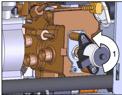
III. 78: Afmonter køleventil 1
